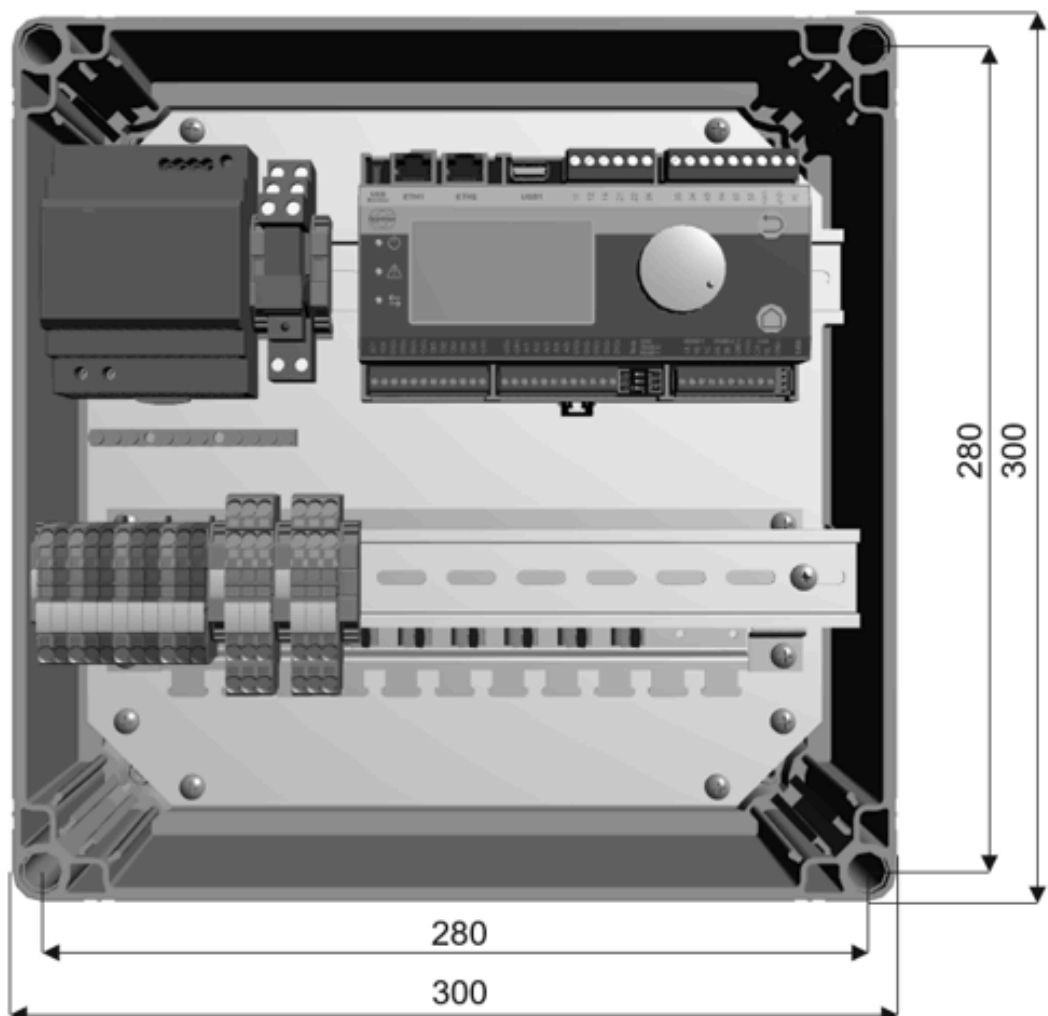
Dimensions du caisson de l'aicore fusion
