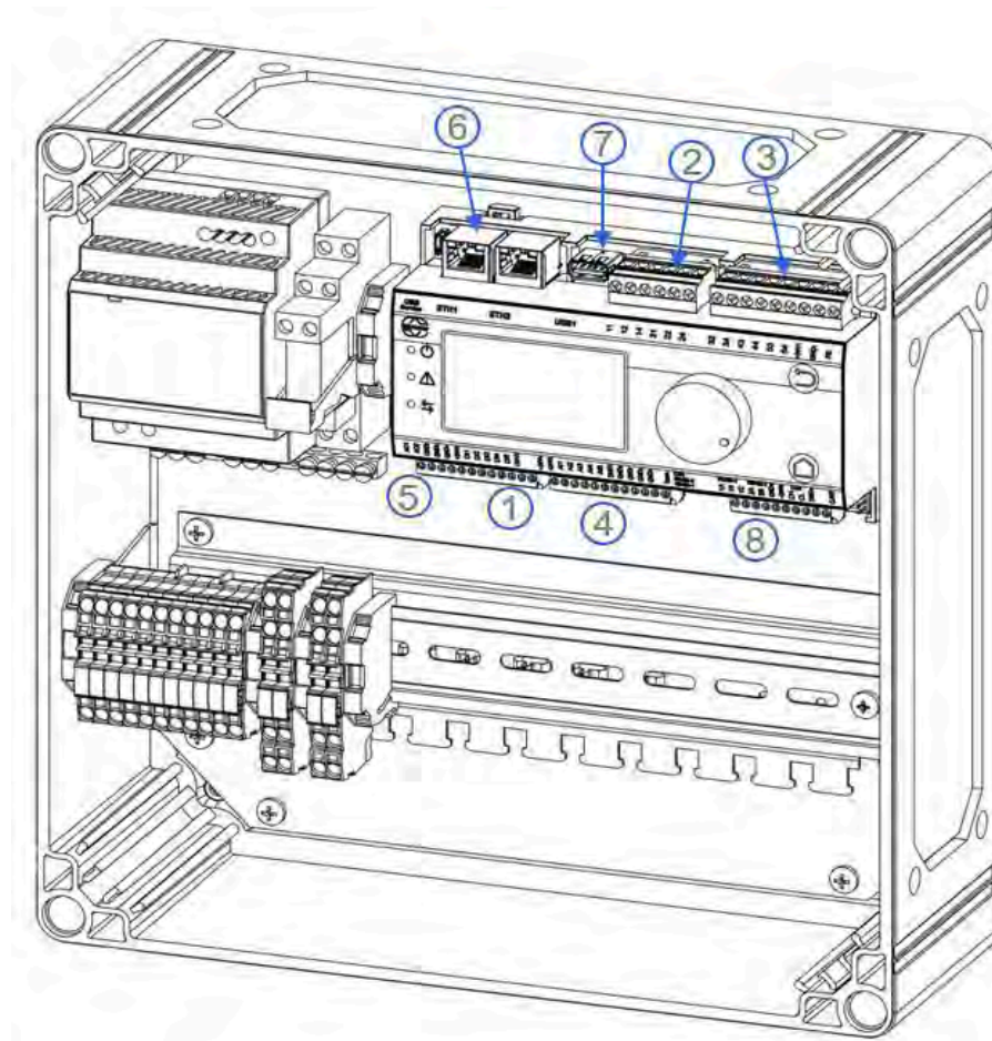
Emplacements des raccordements avec l'aicore fusion
